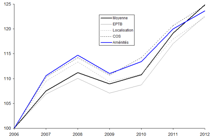
Graphique 1 : Indices de prix, selon les variables explicatives prises en compte
