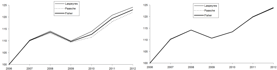
Graphique 2 : Indices de Laspeyres, Paasche et Fisher pour un bien de référence
